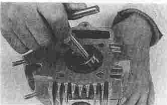
Fig. 41 Klepzitting frezen
