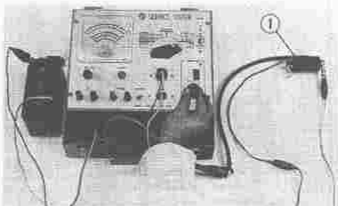
Fig. 108 Ontstekingsspoel test (bobine) ① Ontstekingsspoel (bobine)
