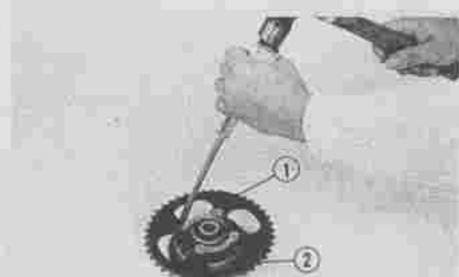
Fig. 78 1) Achterkettingtandwiel 2) Tandwielnaaf
