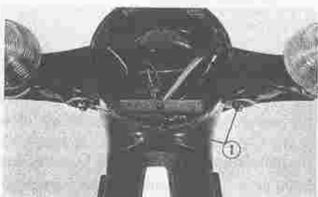
Fig. 89 Demonteren van stuur ① 8 mm bouten C50
