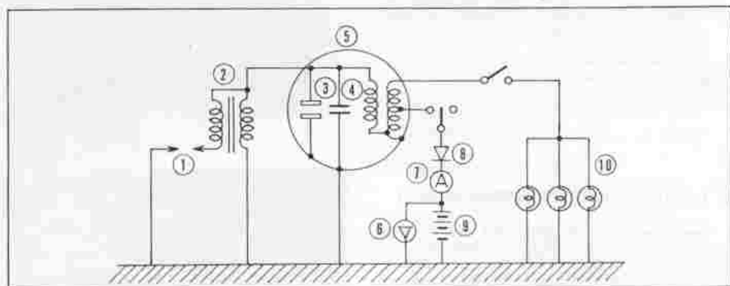
Fig. 104 ① Bougie ② Bobine ③ Onderbreker ④ Condensator ⑤ Vliegwiél-Dynamo ⑥ Voltmeter ⑦ Ampèremeter ⑧ Seleniumgelijkrichter ⑨ Batterij ⑩ Lampen belasting
