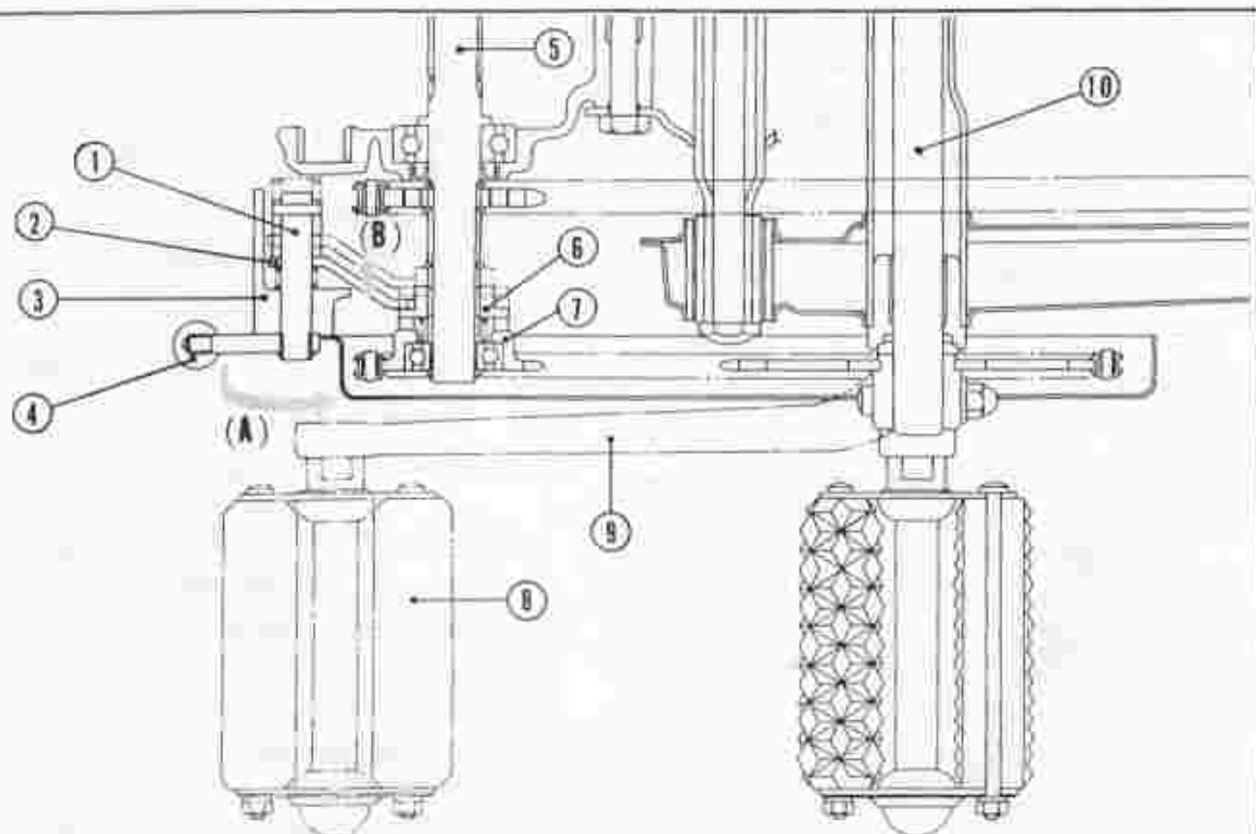
Fig. 99 Schakel systeem
