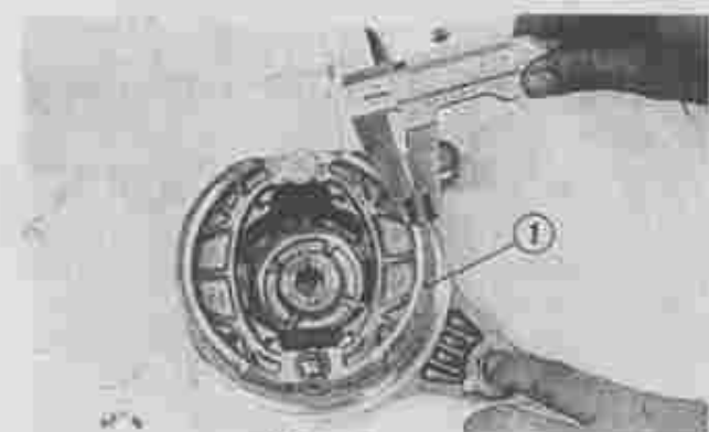
Fig. 80 Meten van remschoenen 1) Remschoen voering
